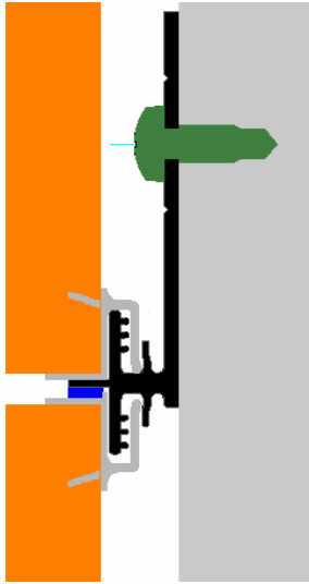
KESİT DETAYI
