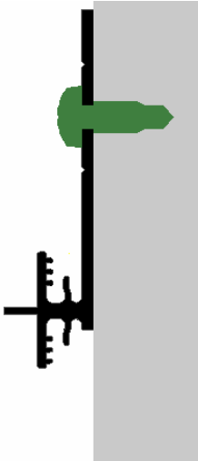
KESİT DETAYI
