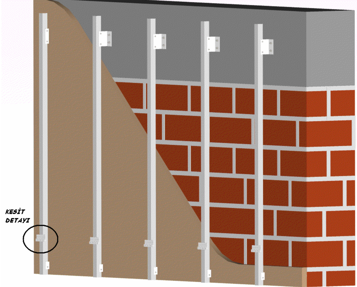
KESİT DETAYI
