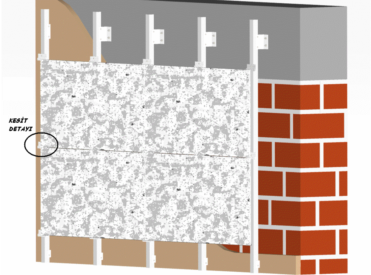
KESİT DETAYI
