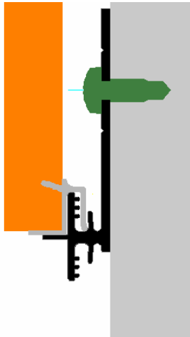
KESİT DETAYI
